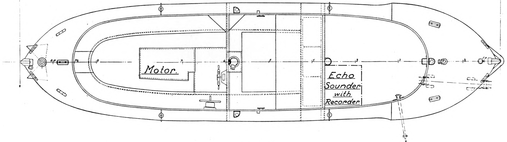
PLAN N° 31
